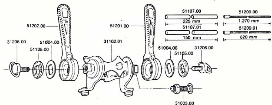
21200.00 Doble mando ZEUS Gran Sport ZEUS double derailleur control lever Gran Sport
