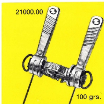
21000.00 Doble mando ZEUS-2000 ZEUS-2000 double derailleur control lever
