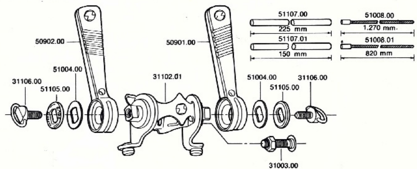
21200.00 Doble mando ZEUS Gran Sport ZEUS double derailleur control lever Gran Sport
